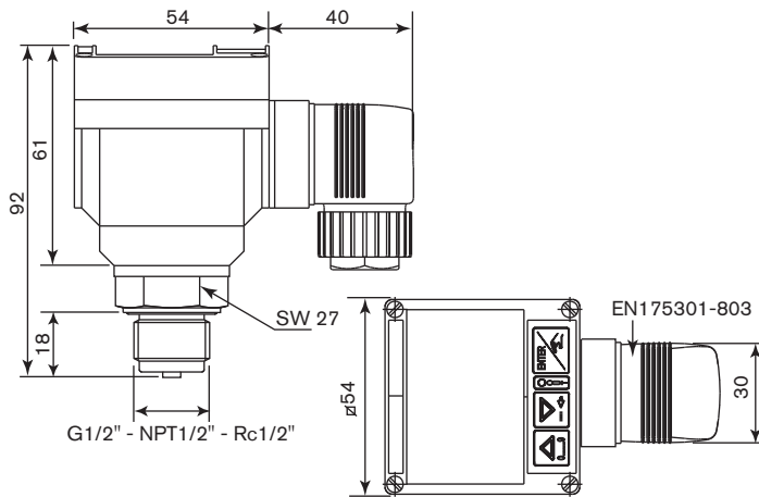
Transmitter EN 175301-803 plug
