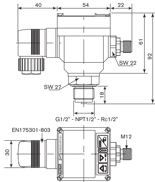
Transmitter / Switch M12 & EN 175301-803 plugs
